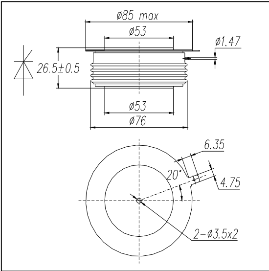
外型图 Outline
