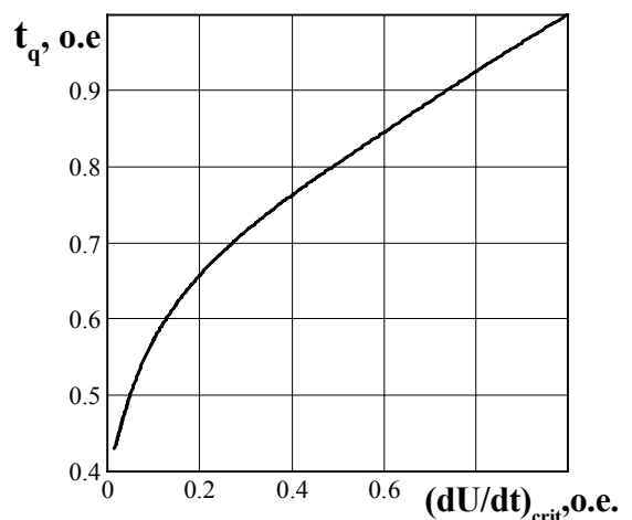
Рисунок 16 - Зависимость времени выключения t_q (о.е.) от скорости нарастания напряжения в открытом состоянии dU_D/dt при T_{im} = 125 \text{ }^\circ\text{C} ; I_T = I_{T(AV)} ; U_D = 0,67 U_{DRM} ; U_R = 100 \text{ В} ; (di/dt)_f = 5 \text{ A/мкс}
