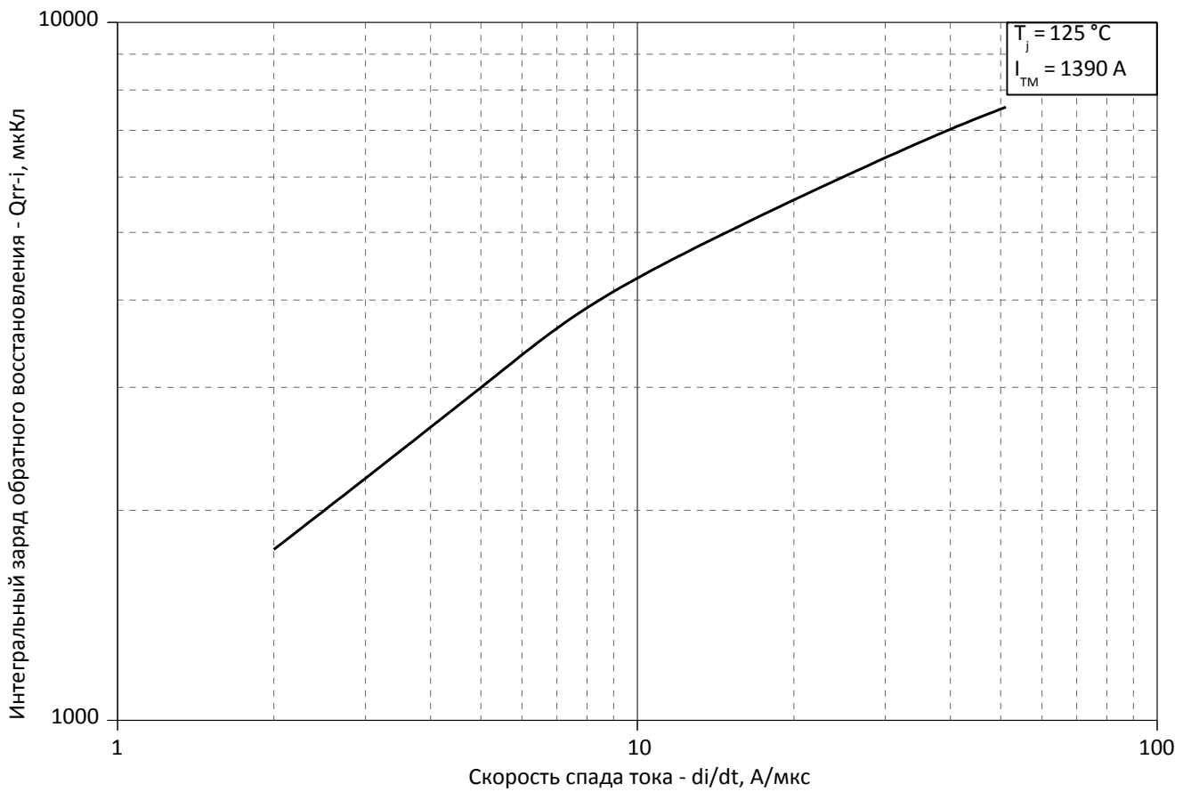
Рис. 3 – Зависимость максимального интегрального заряда обратного восстановления Q_{gr-i} от скорости спада тока di_r/dt в открытом состоянии
