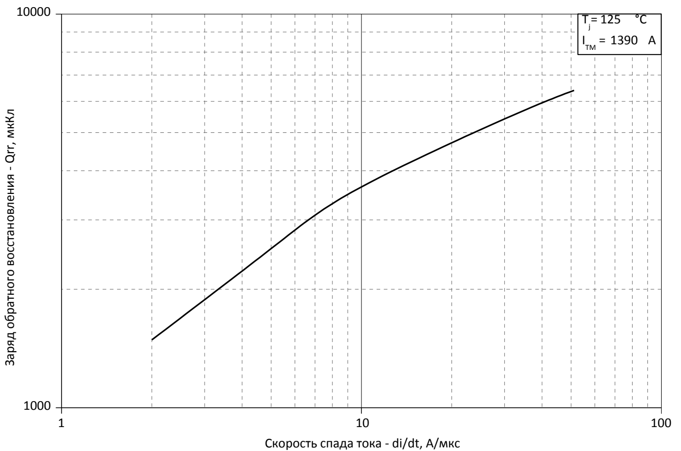
Рис. 4 – Зависимость максимального заряда обратного восстановления Q_{gr} от скорости спада тока di_r/dt (по ГОСТ 24461, хорда 25%) в открытом состоянии
