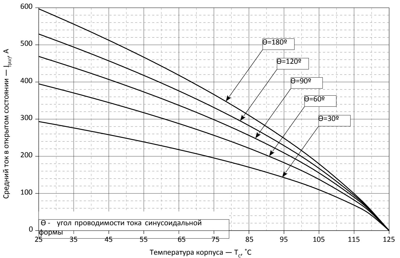
Рис. 9 – Зависимость среднего тока в открытом состоянии I_{TAV} от температуры корпуса T_c для синусоидальной формы тока при различных углах проводимости ( f=50 Гц, Двустороннее охлаждение)
