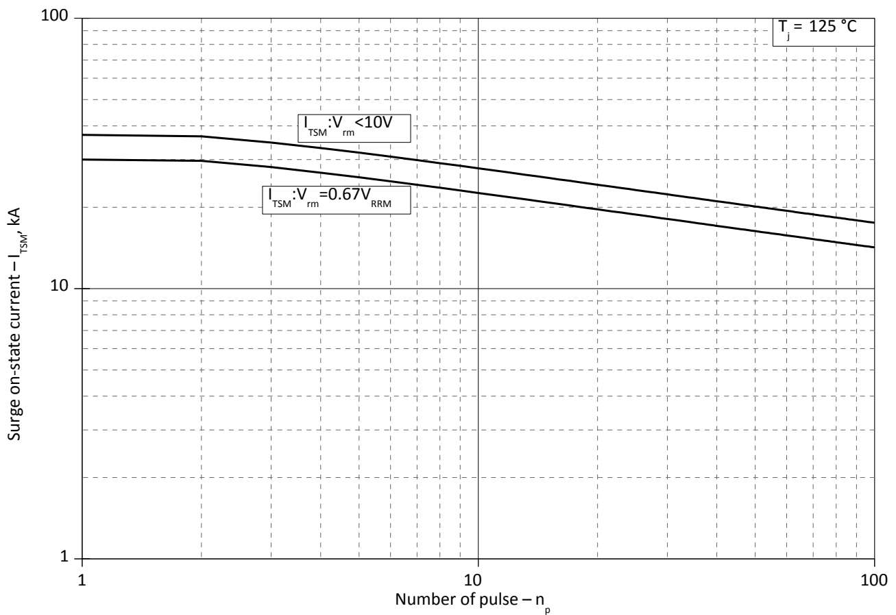
Рис. 12 – Максимальные ударные характеристики
