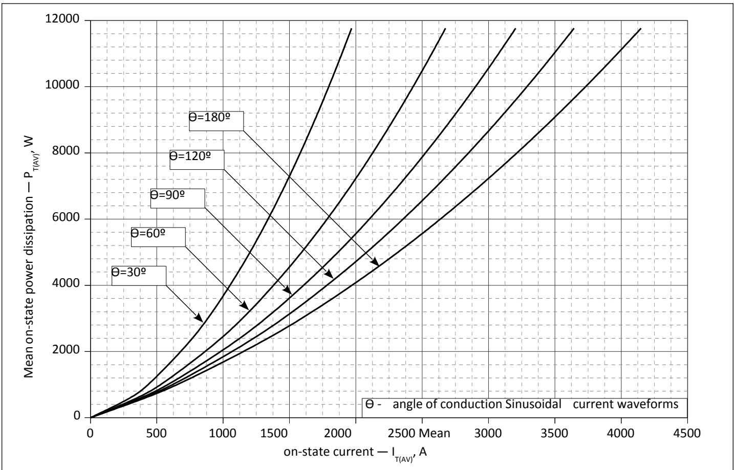
Рис. 7 - Зависимость потерь мощности P_{TAV} от среднего прямого тока I_{TAV} синусоидальной формы при различных углах проводимости ( f=50 Гц, двустороннее охлаждение)
