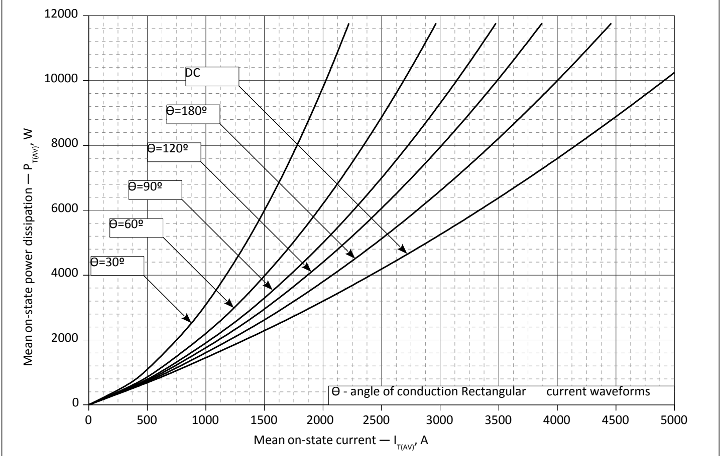
Рис. 8 - Зависимость потерь мощности P_{TAV} от среднего прямого тока I_{TAV} прямоугольной формы при различных углах проводимости ( f=50 Гц, двустороннее охлаждение)
