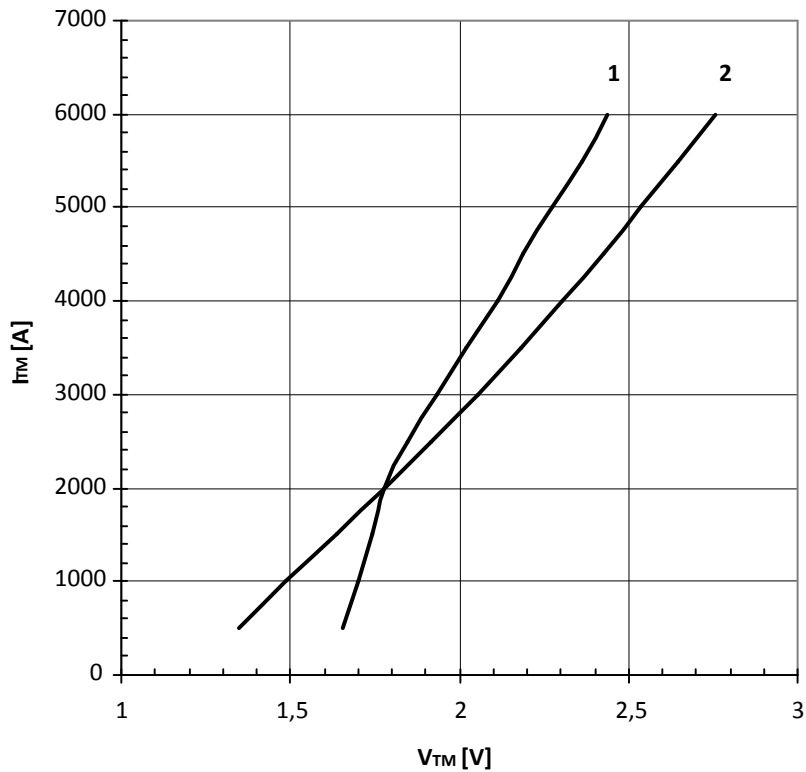
Рис.1 – Предельная вольт-амперная характеристика. 1 – T_j=25\text{ }^{\circ}\text{C} 2 – T_j=125\text{ }^{\circ}\text{C}
