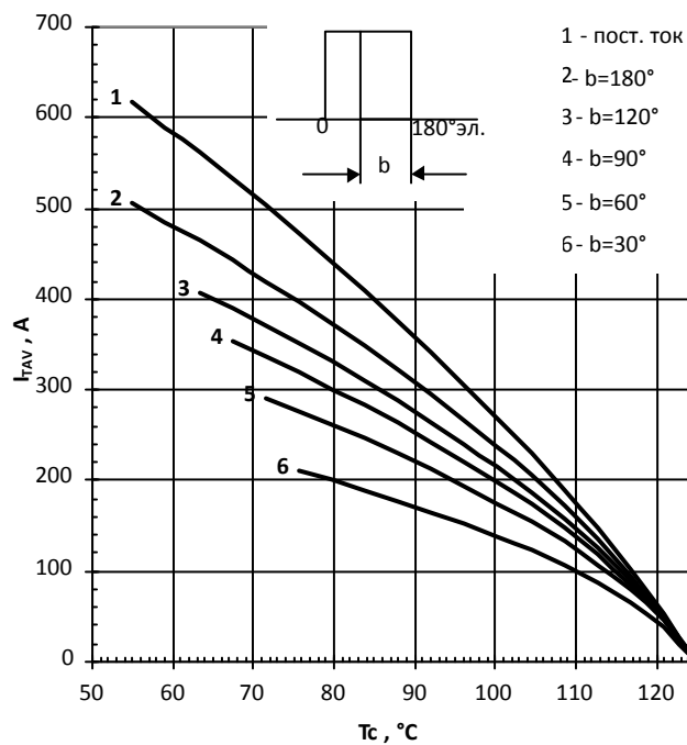
Рис. 3 – Зависимость максимально допустимого среднего тока в открытом состоянии I_{TAV} от температуры корпуса T_c для прямоугольной формы тока при различных углах проводимости, f=50 Гц.
