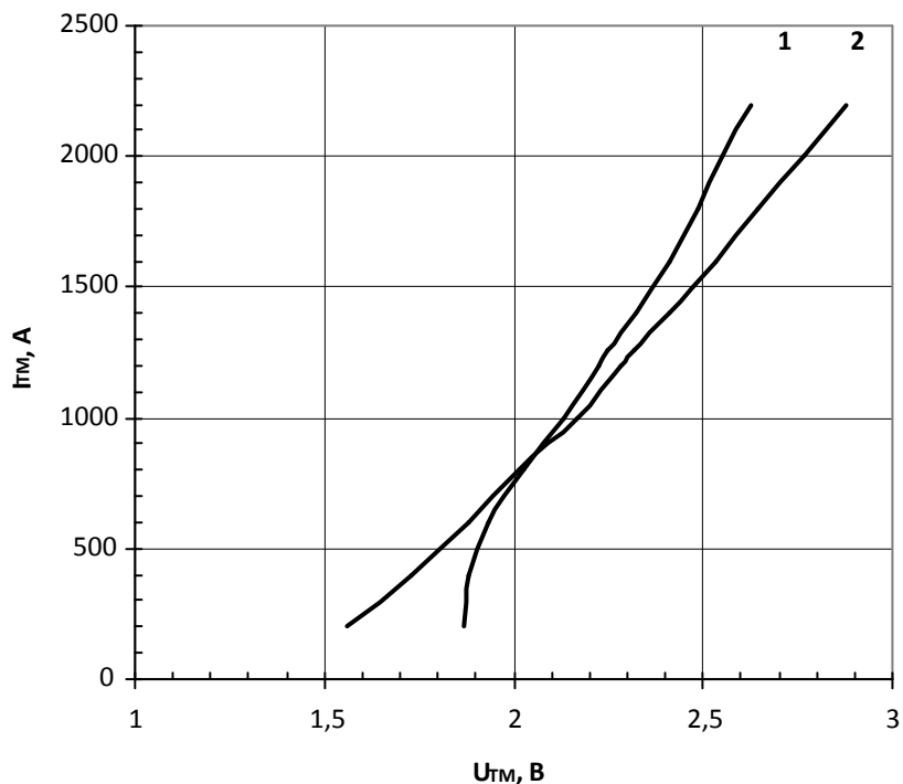
Рис.1 – Предельная вольт-амперная характеристика. 1 – T_j=25\text{ }^\circ\text{C} 2 – T_j=125\text{ }^\circ\text{C}
