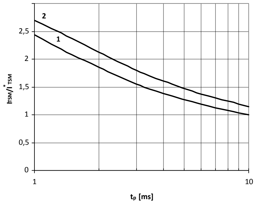
Рис. 28 – Зависимость ударного тока I_{TSM} от длительности импульса t_p для полусинусоидального импульса
