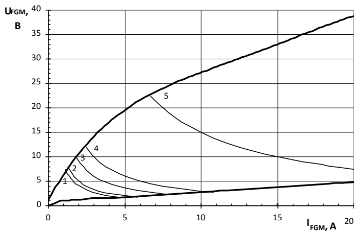
Рис.1 – Предельная вольт-амперная характеристика.
