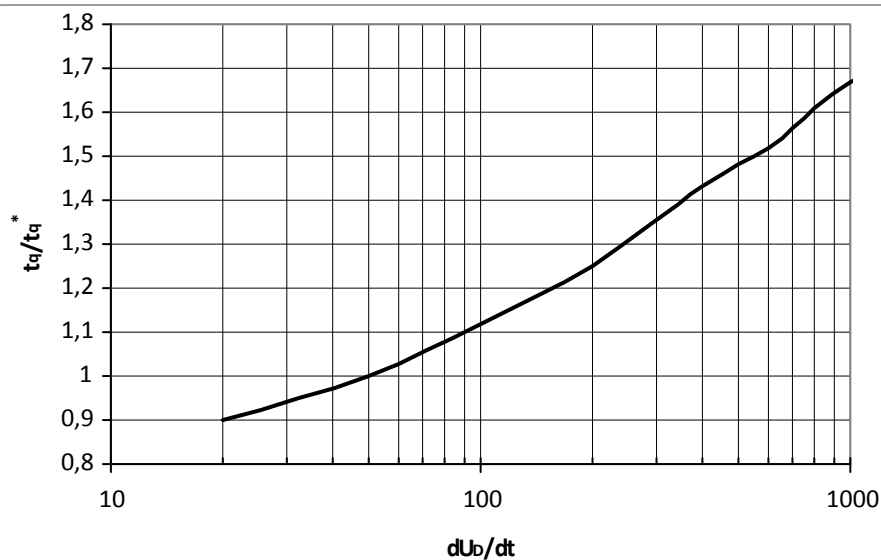
Рис. 6 — Зависимость времени выключения t_q от скорости нарастания напряжения du_b/dt
