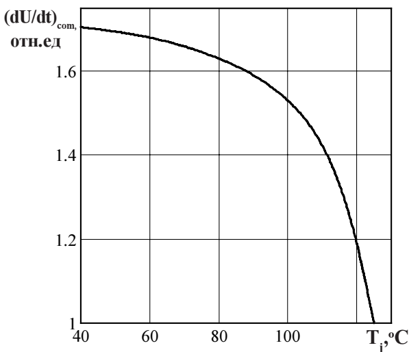
Рисунок 12 - Зависимость критической скорости нарастания коммутационного напряжения (dU_D/dt)_{com} (отн.ед.) от температуры структуры T_j ^\circ\text{C} при I_T = I_{TRMS} , t_i = 10\text{ мс} .
