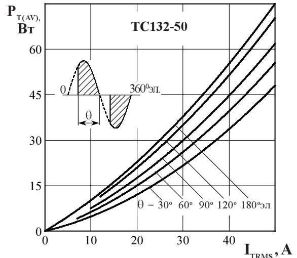
Рисунок 4 - Зависимость средней мощности потерь P_{T(AV)} от действующего значения тока I_{TRMS} в открытом состоянии синусоидальной формы частоты f = 50 Гц
