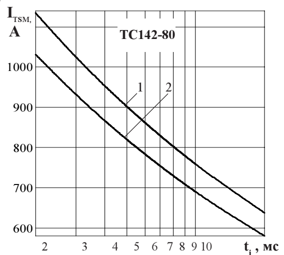
Рисунок 5 - Зависимость допустимой амплитуды ударного тока в открытом состоянии I_{TSM} от длительности импульса тока t_i при исходной температуре структуры T_j = 25^\circ C (1) и максимальной температуре T_{jm} (2)
